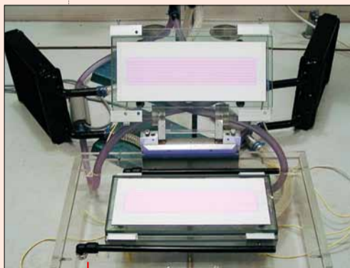
Speciální přístroj na povrchovou úpravu plošných materiálů plazmatem, který vyvinul kolektiv profesora Mirko Černáka. Foto: Archiv M. Černáka.
